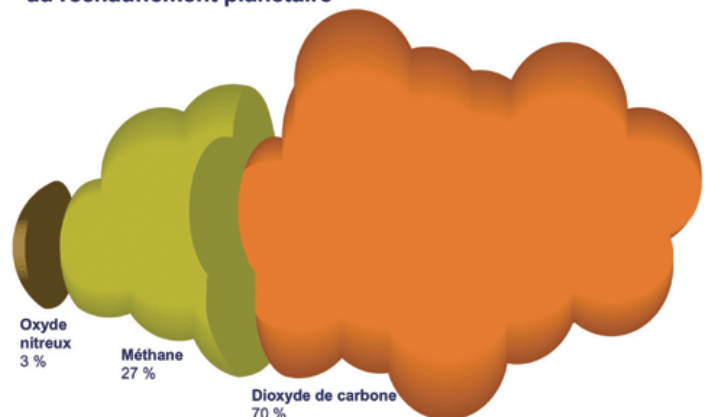
Contribution des actuels gaz à effet de serre au réchauffement planétaire
