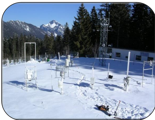
Station météo au Col de Porte, Chartreuse
